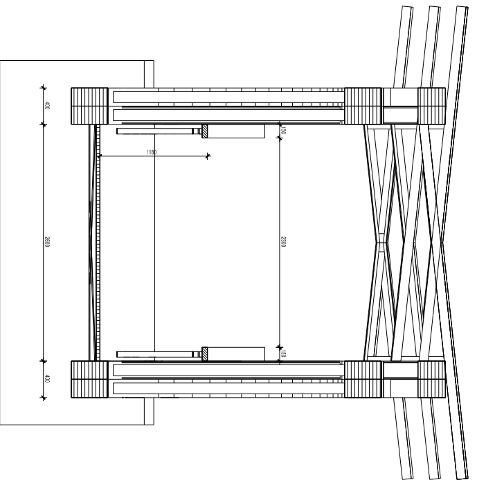
COUPE 1/20
