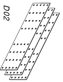
JOINT DE MONTAGE 1/10
