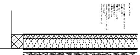
1.2 PAROI BOIS BARDEE : bardage horizontal
