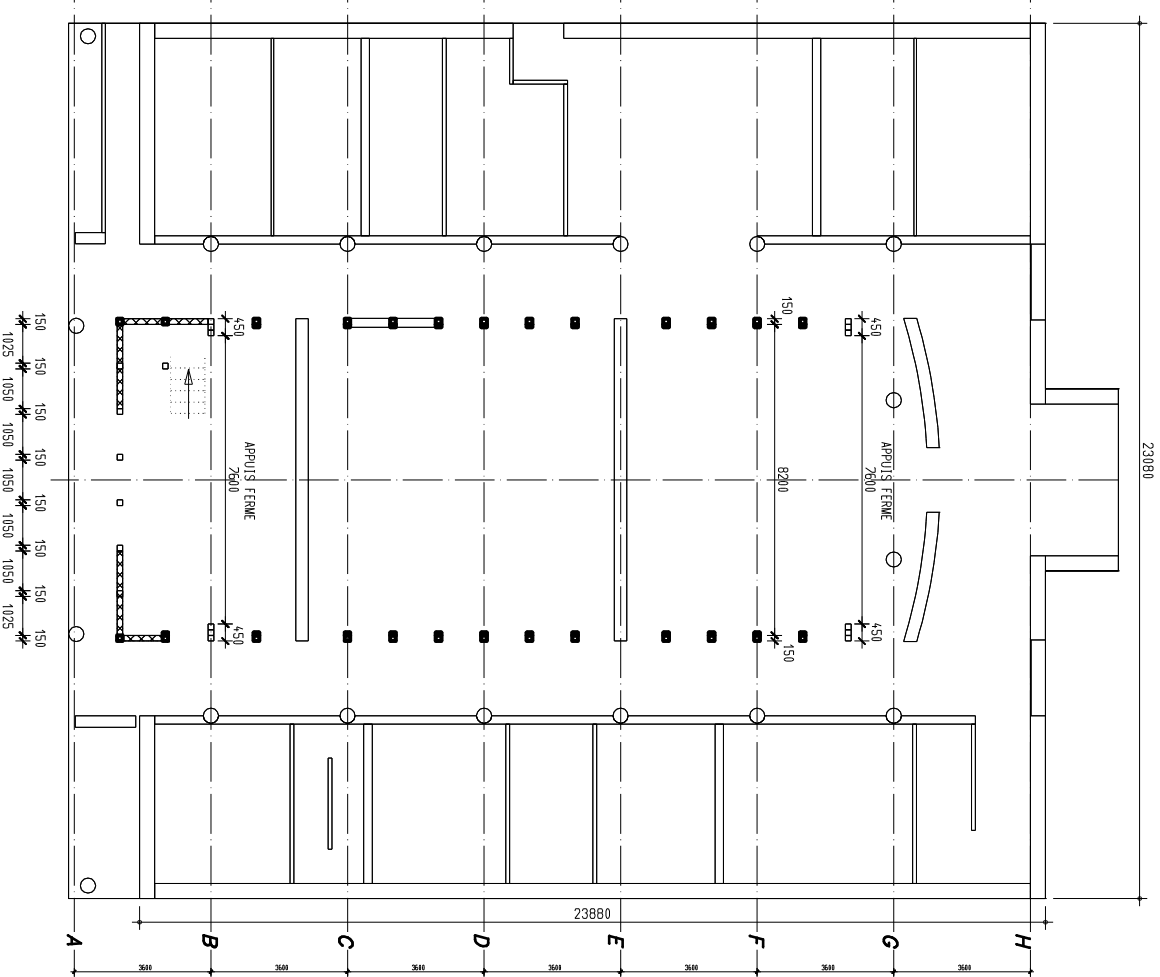
PLAN D'IMPLANTATION 1/100 TRAME 1200 mm , SAUF MENTION
